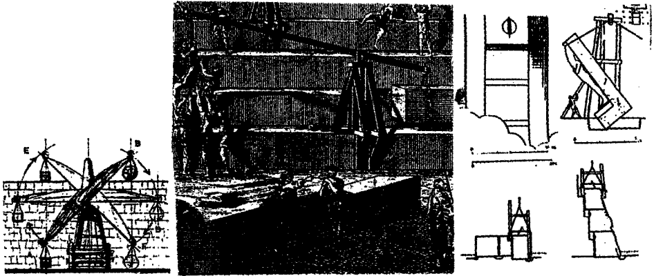
(شكل : ١٦) رسوم تخيلية لآلات رافعة يرجح إستخدامها من قبل المصري القديم لرفع الكتل الحجرية لمستويات مختلفة بالمقابر الهرمية - دولة قديمة أ- و
